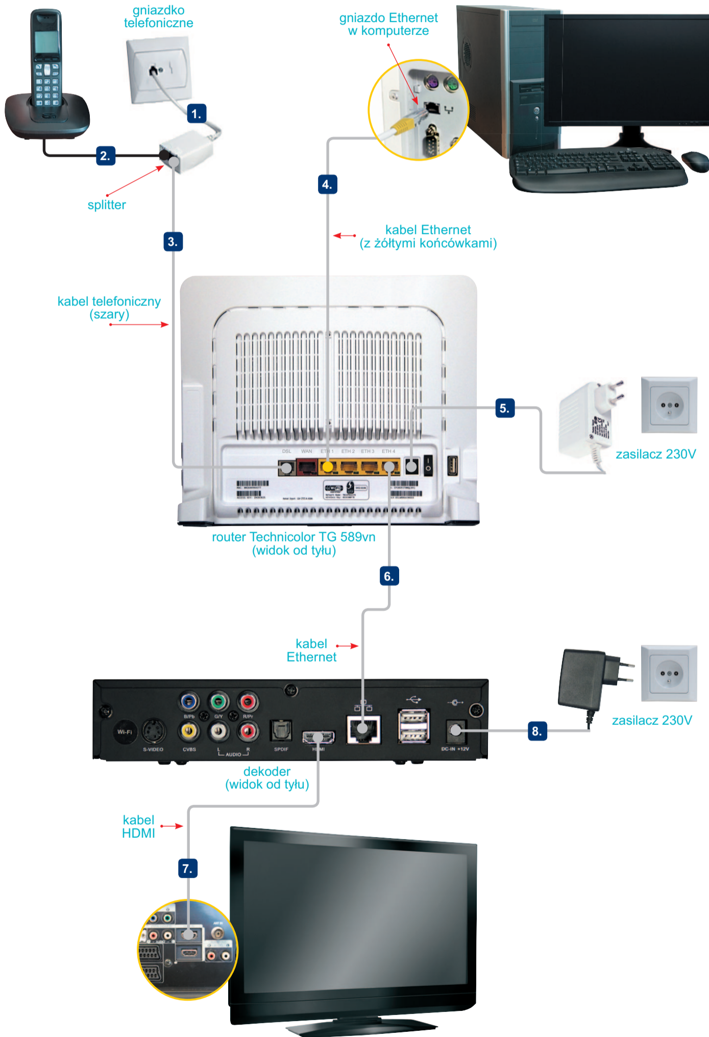
PHONE – port do podłączenia telefonu ADSL – port do podłączenia routera
