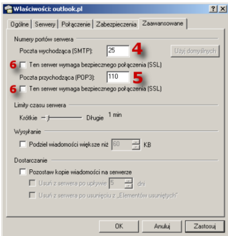
Rys.7. Ustawienia zaawansowane kont pocztowych.
